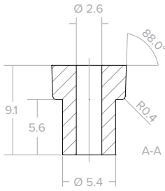
Steatite Grommet
